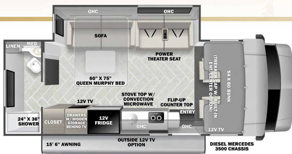
24SRB (Mercedes-Benz Sprinter 3500)
