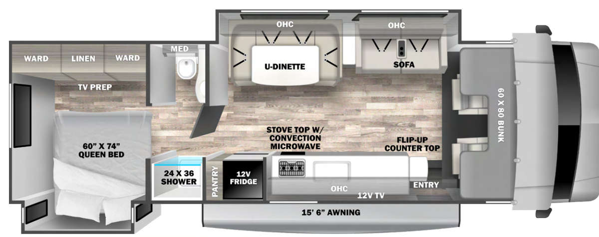
32DSK (Available on Ford E450)
