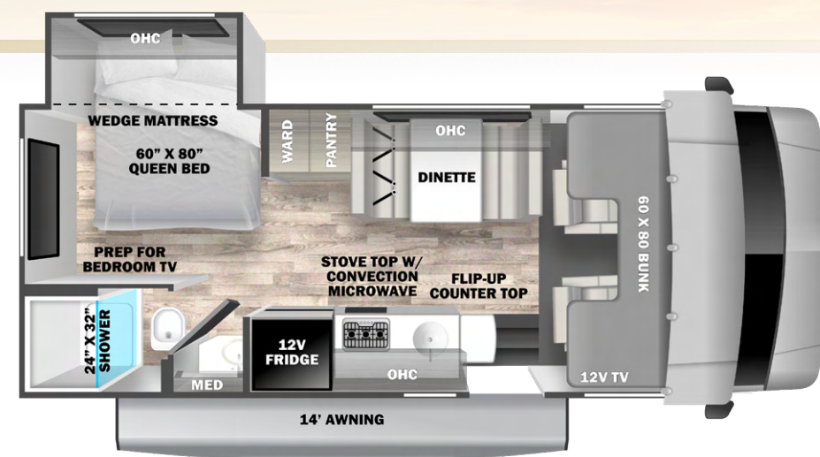
23S (Available on Ford E350/Chevy 3500)
