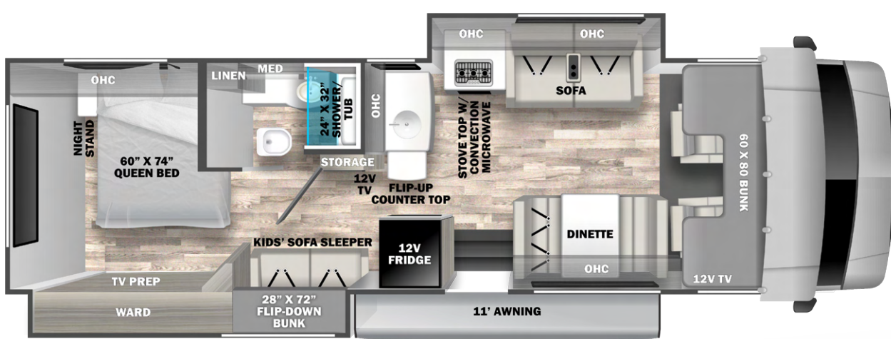
32DSB (Available on Ford E450)
