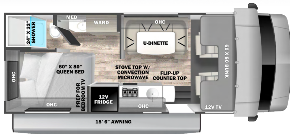
22N (Available on Ford E350/Chevy 3500)
